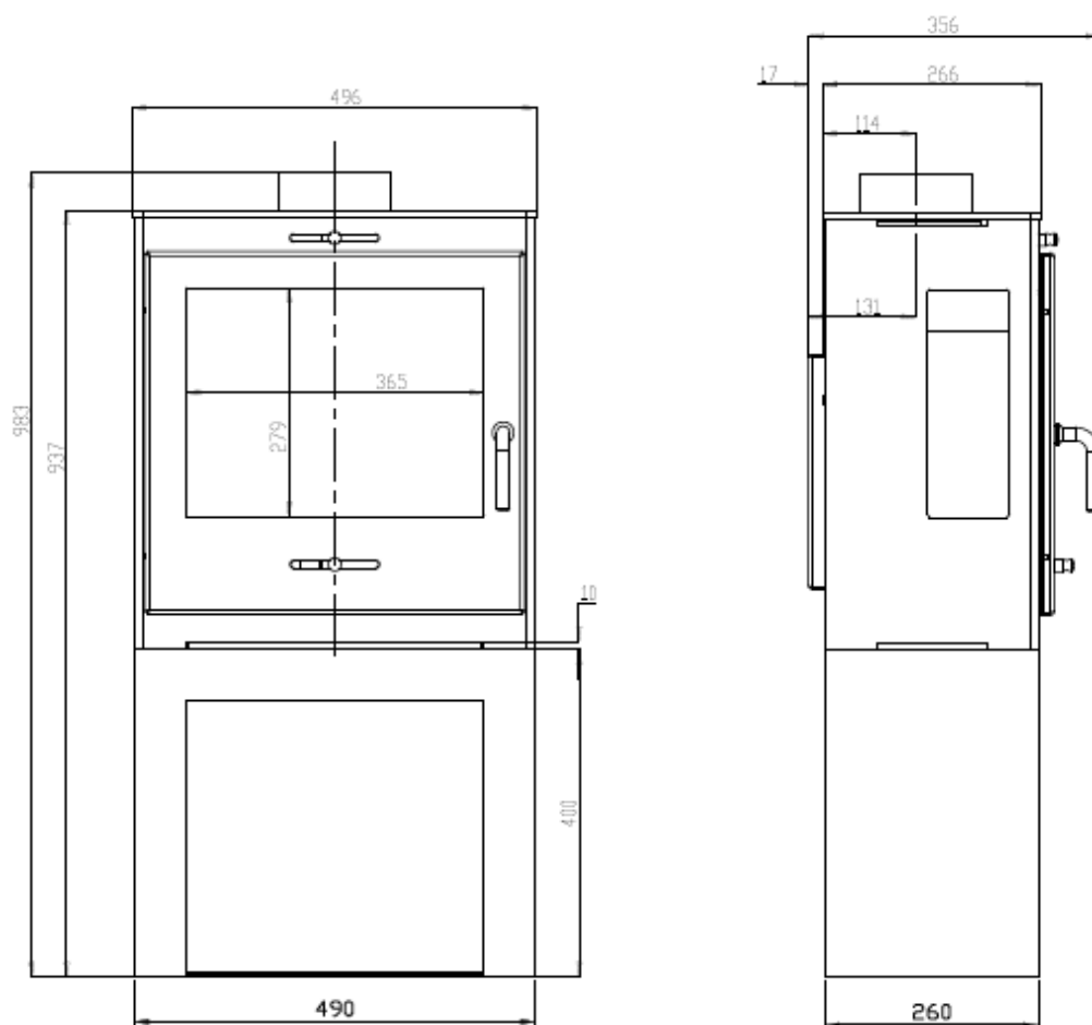
Technický výkres hede 1D Panorama:
