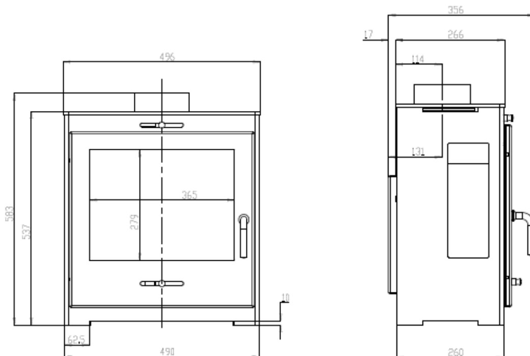
Technický výkres hede 1 Panorama:
